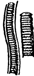
Fig. 4 : Phormidium
