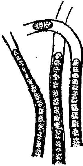
Fig. 3 : Lyngbya
