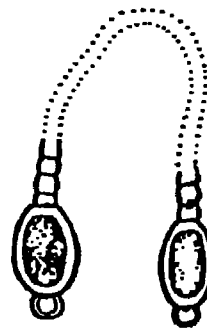
Fig. 6 : Cylindrospermum
