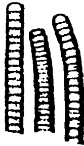
Fig. 2 : Oscillatoria
